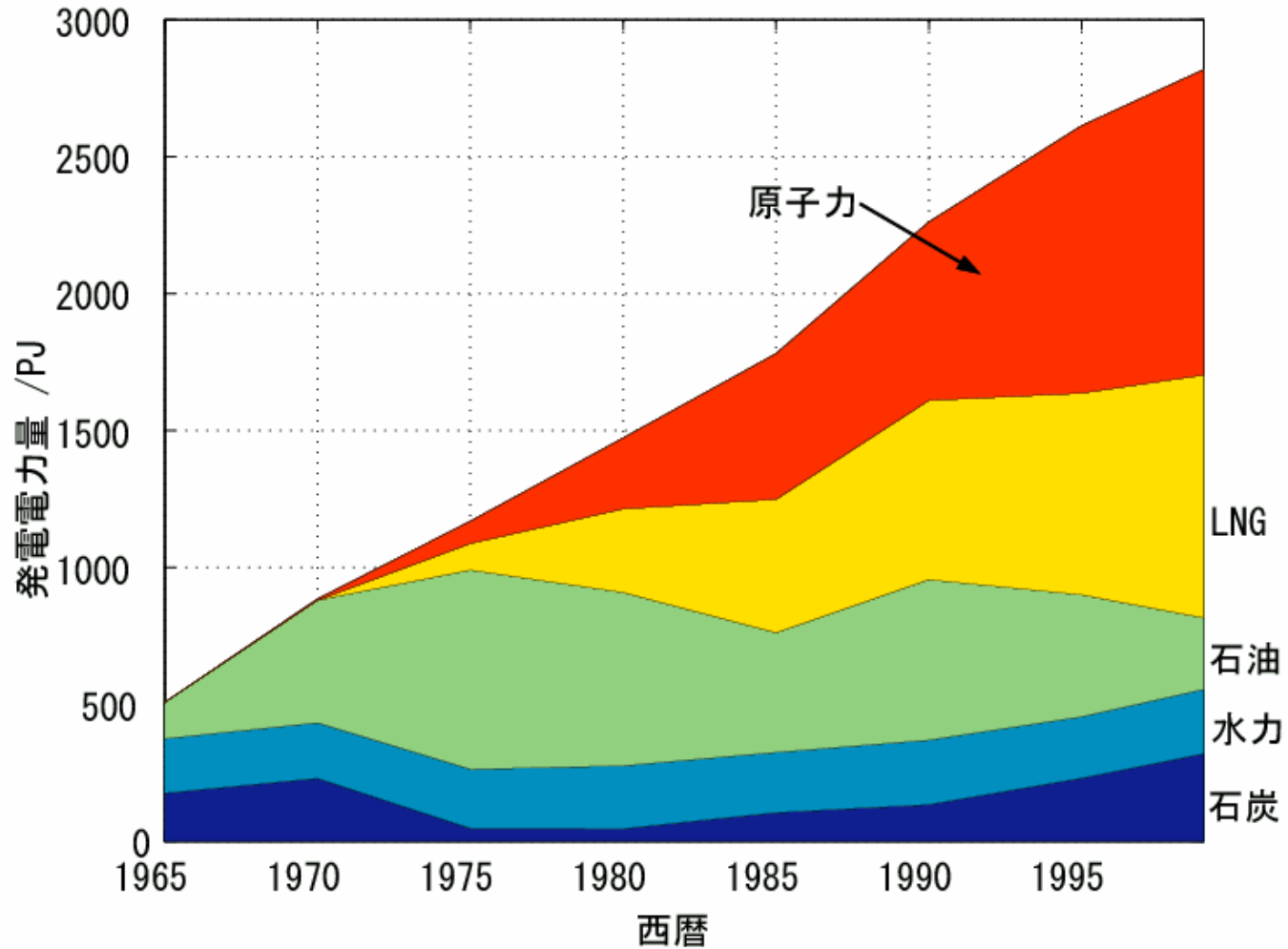
発電電力量の変遷（9電力会社計）
